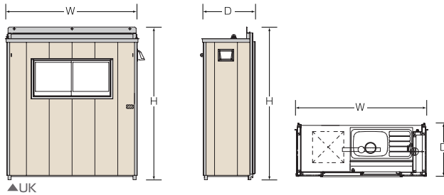
キッチンユニット (UK)
