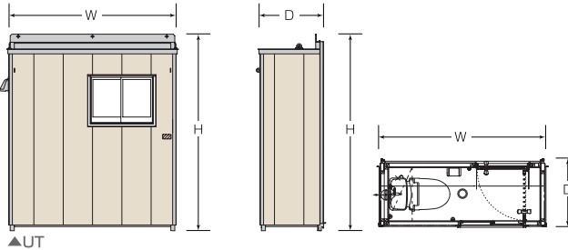
トイレユニット (UT)
