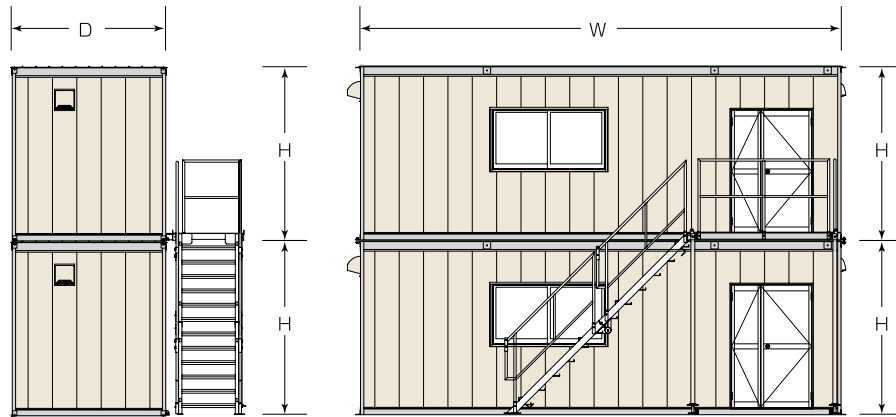
▲RS-50 2階建てタイプ
