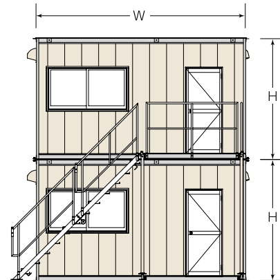
▲RS-30 2階建てタイプ
